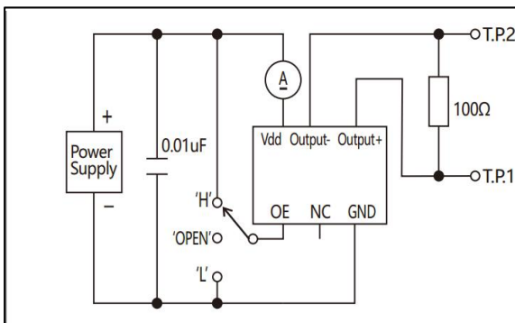
LVDS
