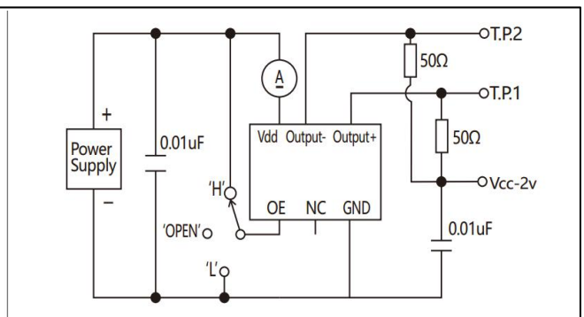
LVPECL
